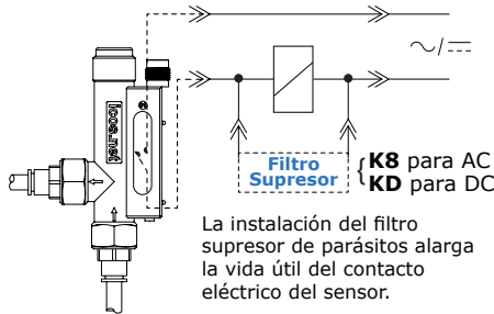
Filtro Supresor K8 para instalación eléctrica (AC) (viene con el producto)
